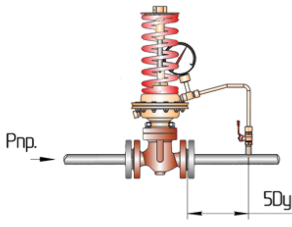
Схема подключения УРРД® НО для регулирования давления «после себя»
